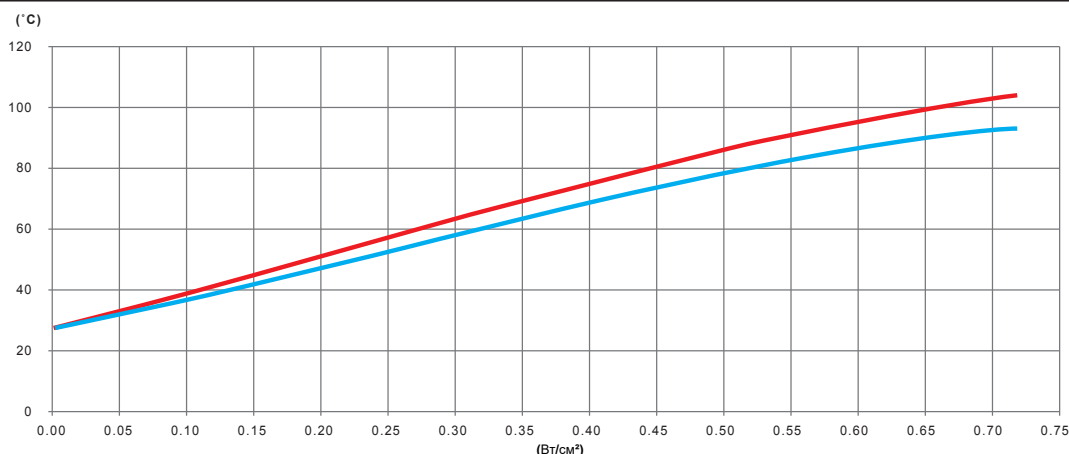
Изменение в зависимости от мощности в Вт/см² силиконовой нагревательной ленты и температуры стенки оцинкованной стальной трубы, заполненной нециркулирующей водой, без теплоизоляции
