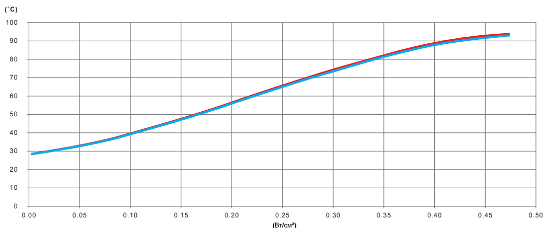
Изменение в зависимости от мощности в Вт/см² силиконовой нагревательной ленты и температуры стенки оцинкованной стальной трубы, заполненной нециркулирующей водой и теплоизолированной 20 мм пеной PVC-NBR
