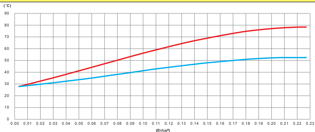
Изменение в зависимости от мощности в Вт/см² силиконовой нагревательной ленты и температуры стенки пустой нетеплоизолированной трубы из PVC
